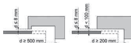
Rysunek 2 - Bezpieczna odległość
