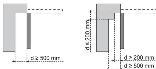
Figuur 4 - Veiligheidsafstand
