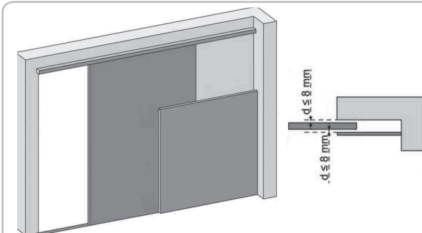
Rysunek 1 - Zabezpieczenie mechaniczne
